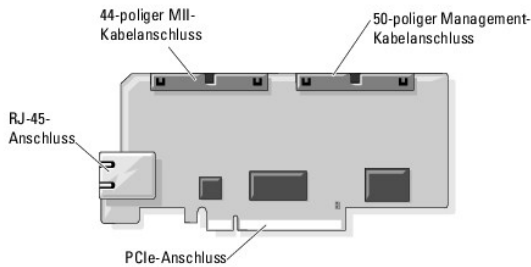
Abbildung 1-1. DRAC 5-Hardwarefunktionen
